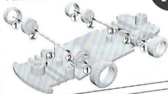
车轮及底部拼装图
