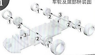
车轮及底部拼装图
